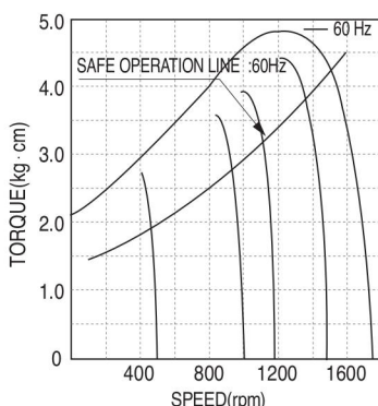
▲ S9I40GA()-V12 S9I40GB()-V12 S9I40GA()-V12(TP) S9I40GB()-V12(TP) S9I40GA()-V12CE S9I40GB()-V12CE
